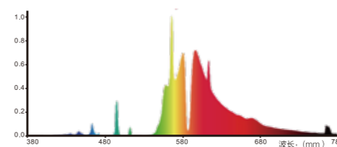
光谱图
