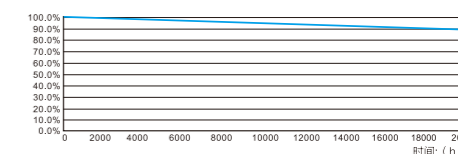
光通维持率
