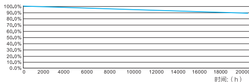
光通维持率
