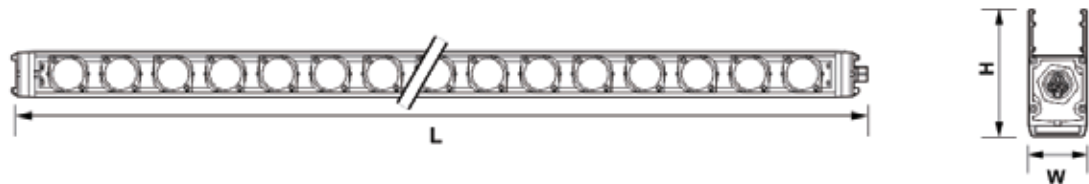
产品尺寸示意图
