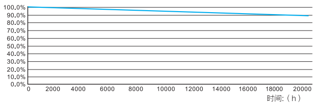
光通维持率
