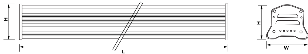
产品尺寸示意图
