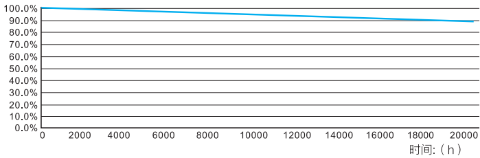
光通维持率
