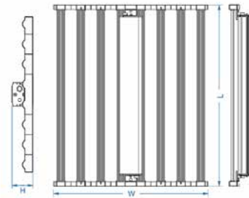
产品尺寸示意图
