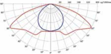
配光曲线
